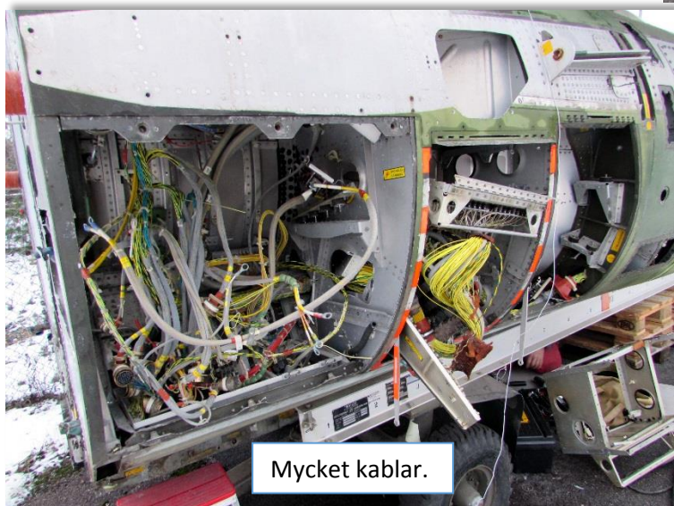
Bortkapad del från 37 Viggen
